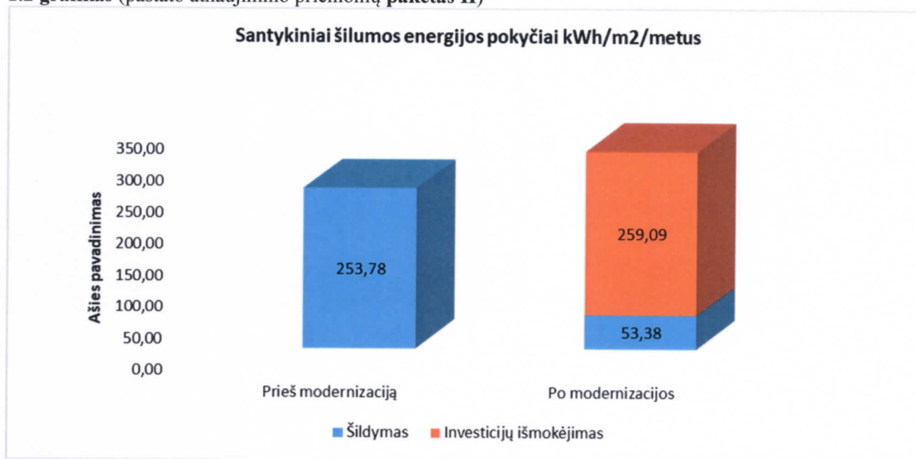
1.2 grafikas (pastato atnaujinimo priemonių paketas II )
