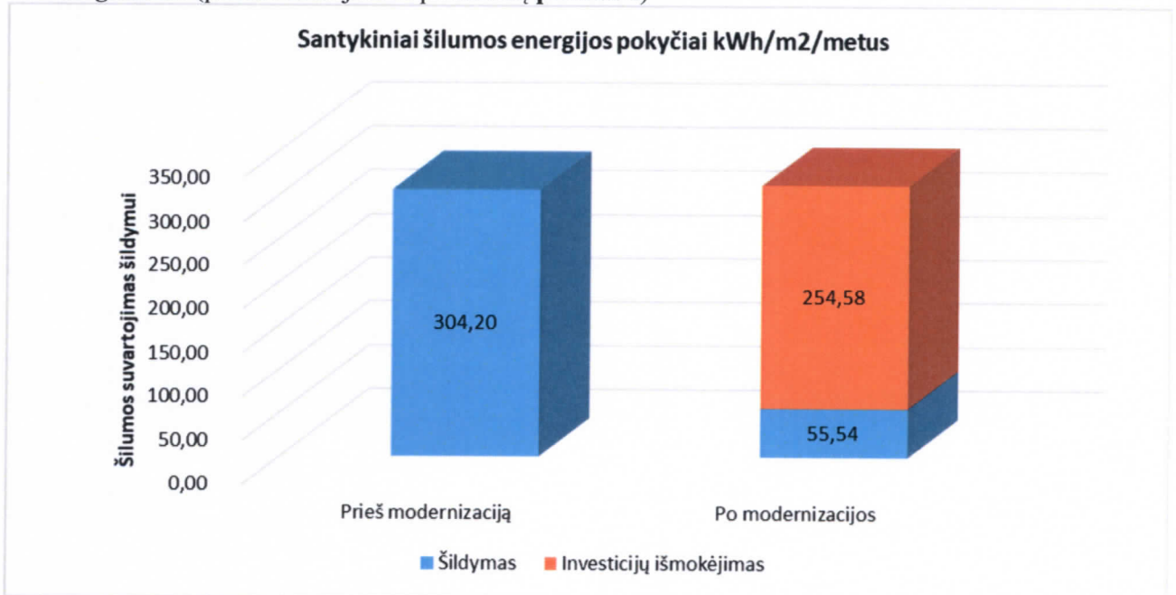
1.1 grafikas (pastato atnaujinimo priemonių paketas I )
